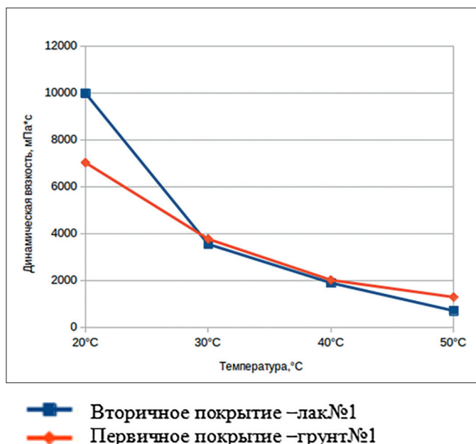
Рис. 1. Зависимость динамической вязкости от температуры для схемы покрытий №1
