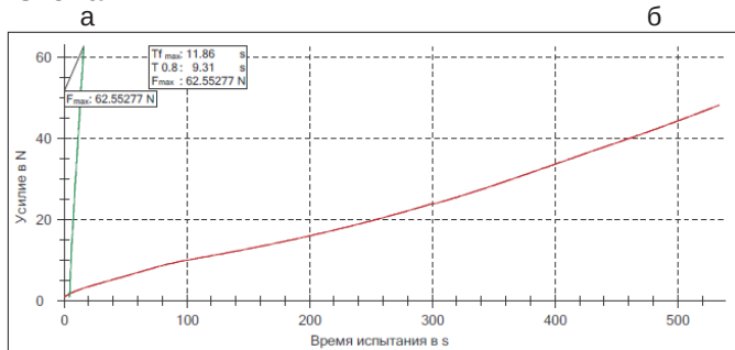
Рис. 3. Прочность на разрыв полимерного покрытия с оптического волокна для схем покрытий №1,2,3,4 при скорости сдвиговых усилий: б-10 м/мин; а-500 м/мин
