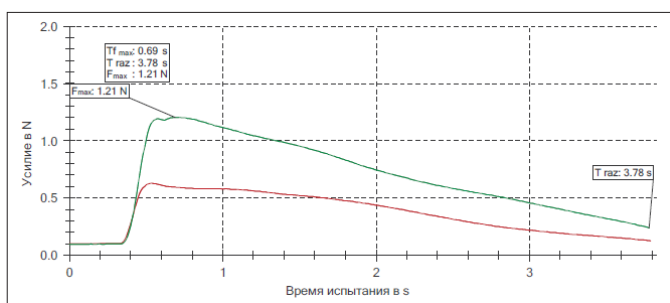
Рис. 4. Усилия снятия полимерного покрытия с оптического волокна для схем покрытий №1,2,3,4
